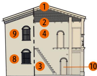
剖面圖
